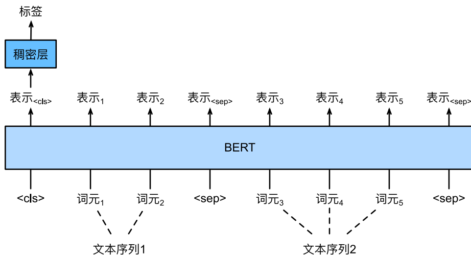
图15.6.2: 文本对分类或回归应用程序的BERT微调，如自然语言推断和语义文本相似性（假设输入文本对分别有两个词元和三个词元）
