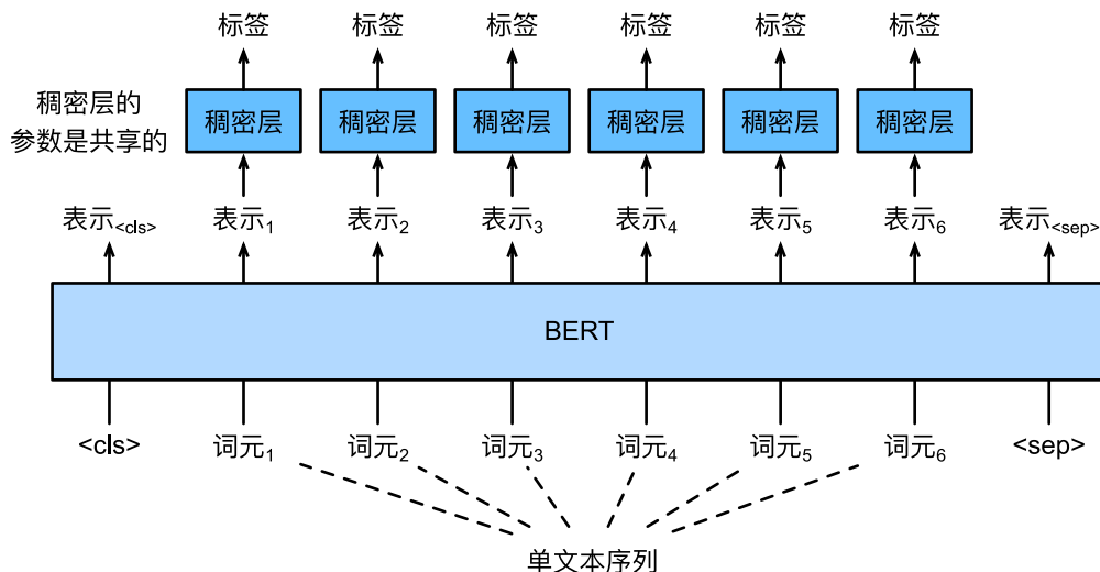
图15.6.3: 文本标记应用的BERT微调，如词性标记。假设输入的单文本有六个词元。
