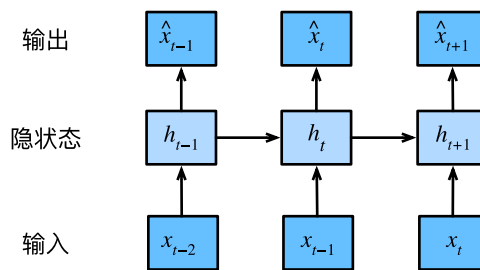
图8.1.2: 隐变量自回归模型
