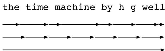
图8.7.1: 比较RNN中计算梯度的策略，3行自上而下分别为：随机截断、常规截断、完整计算
