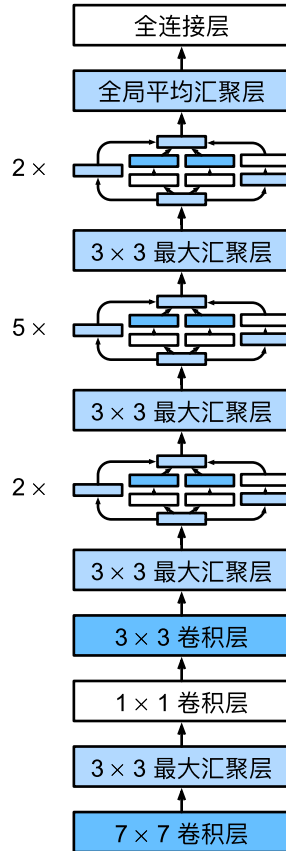
图7.4.2: GoogLeNet架构。
