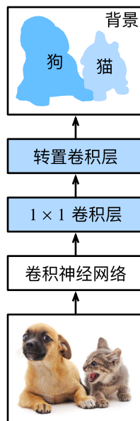
图13.11.1: 全卷积网络
