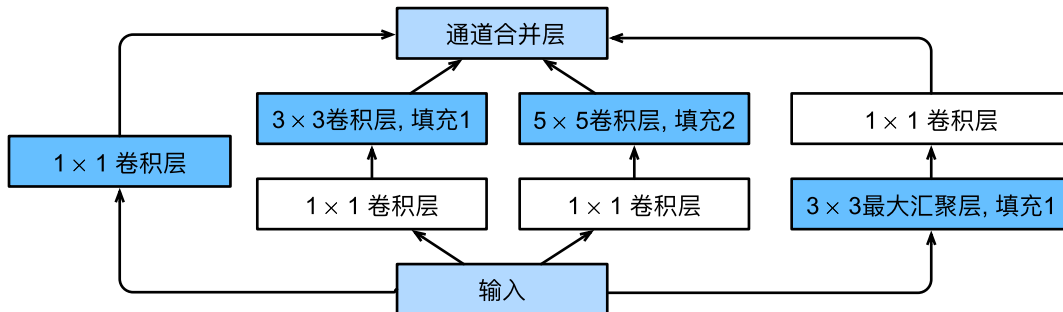
图7.4.1: Inception块的架构。
