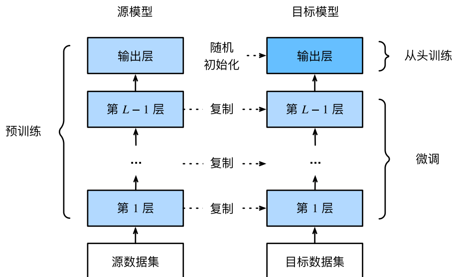
图13.2.1: 微调。
