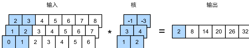
图15.3.3: 具有3个输入通道的一维互相关运算。阴影部分是第一个输出元素以及用于输出计算的输入和核张量元素： 2 \times (-1) + 3 \times (-3) + 1 \times 3 + 2 \times 4 + 0 \times 1 + 1 \times 2 = 2
